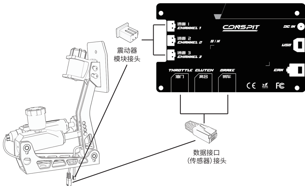
接头图示
