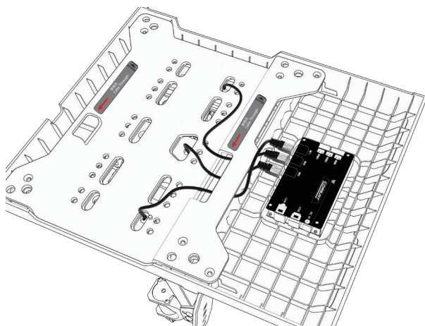
数据线连接示意图
