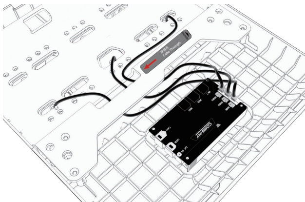
震动模块连接示意图
