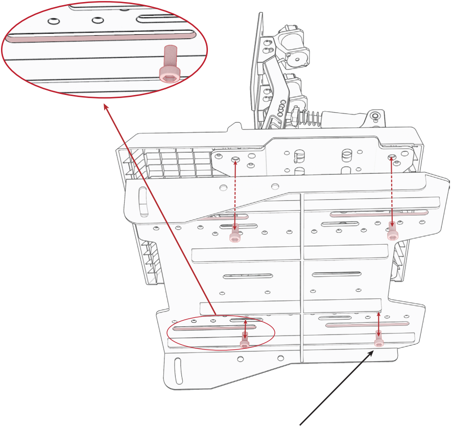
M8*16mm 杯头内六角螺栓 (4 颗)
